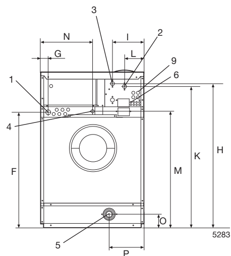
Achterzijde
