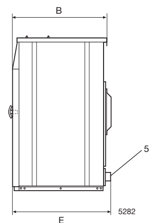
Rechts, zijkant
